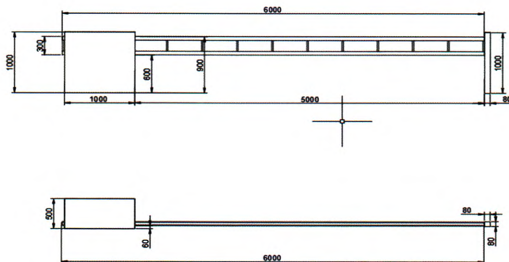
Рис. 2. Габаритные размеры
